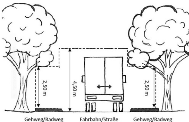
Bild: Lichtraumprofil
